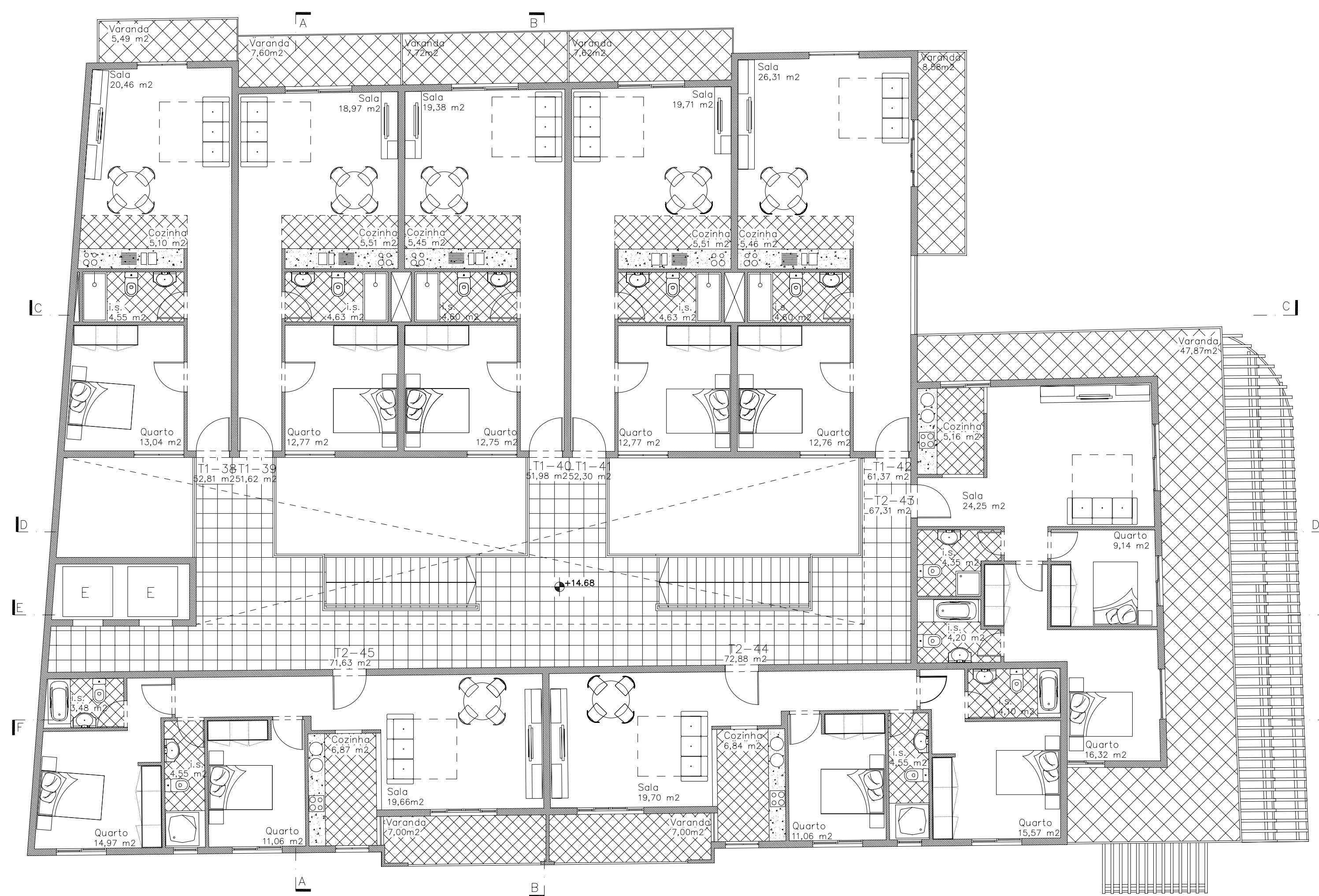
Planta Baixa do 5º Andar Esc. 1:100
