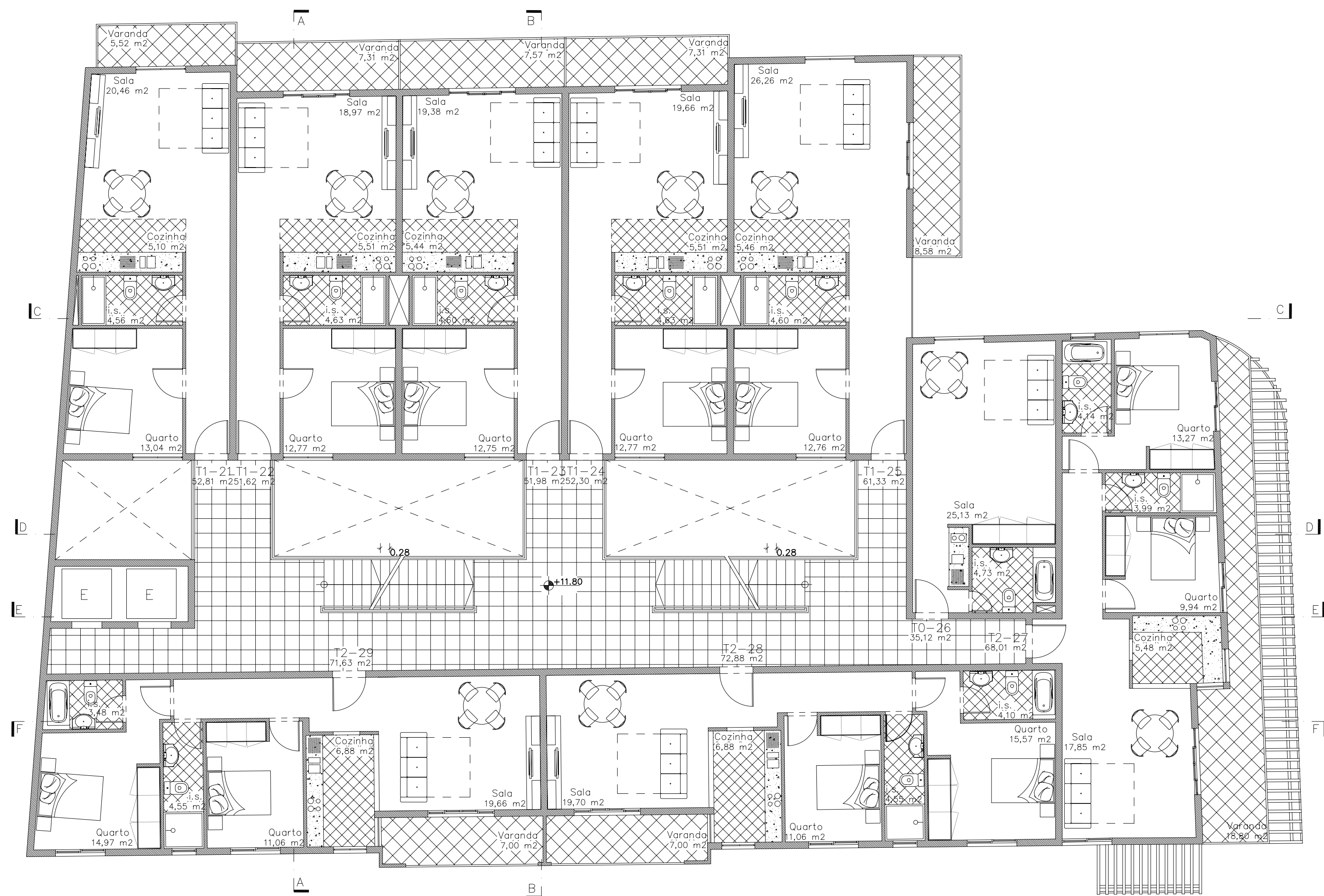
Planta Baixa do 3º Andar Esc. 1:100
