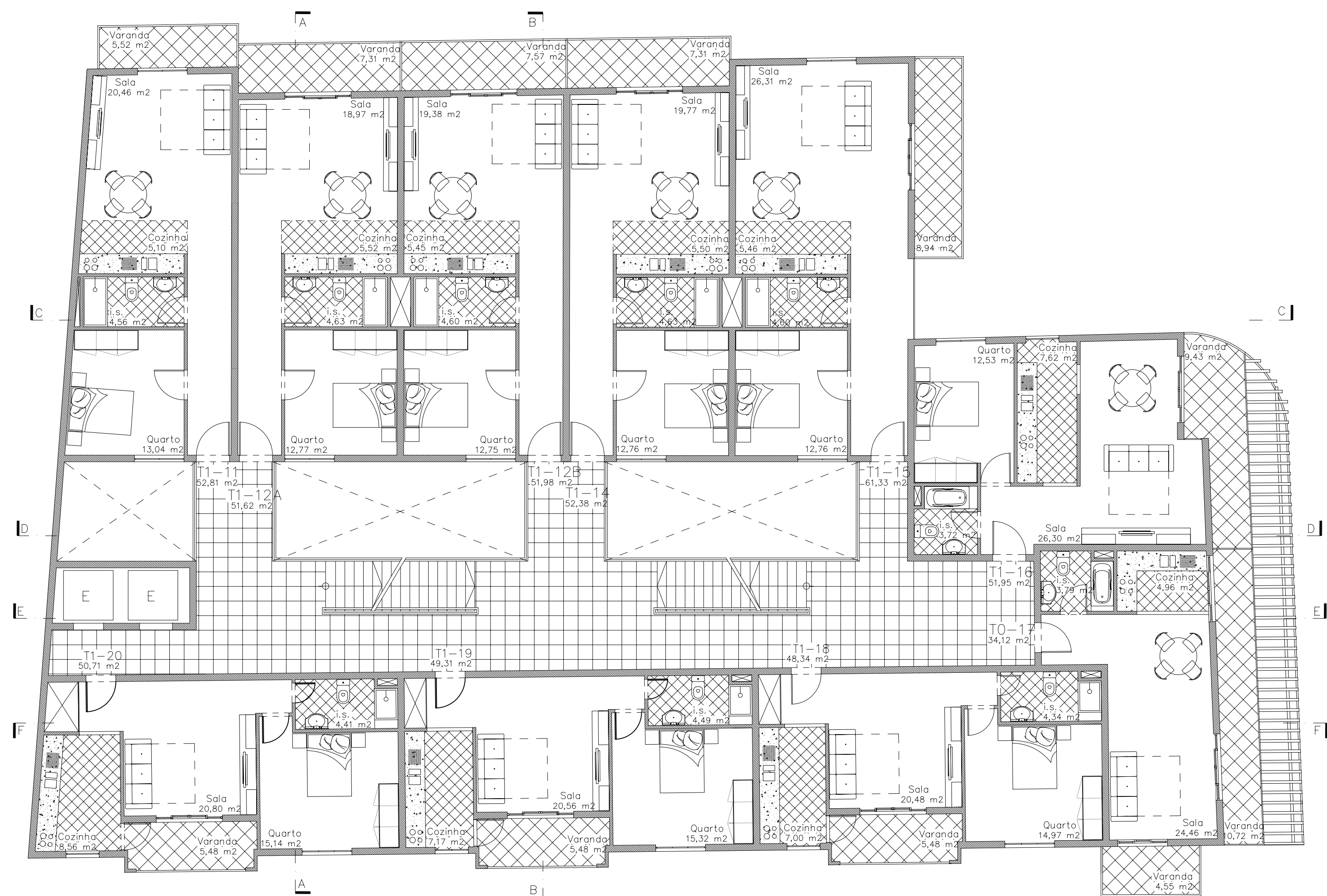
Planta Baixa do 2º Andar Esc. 1:100
