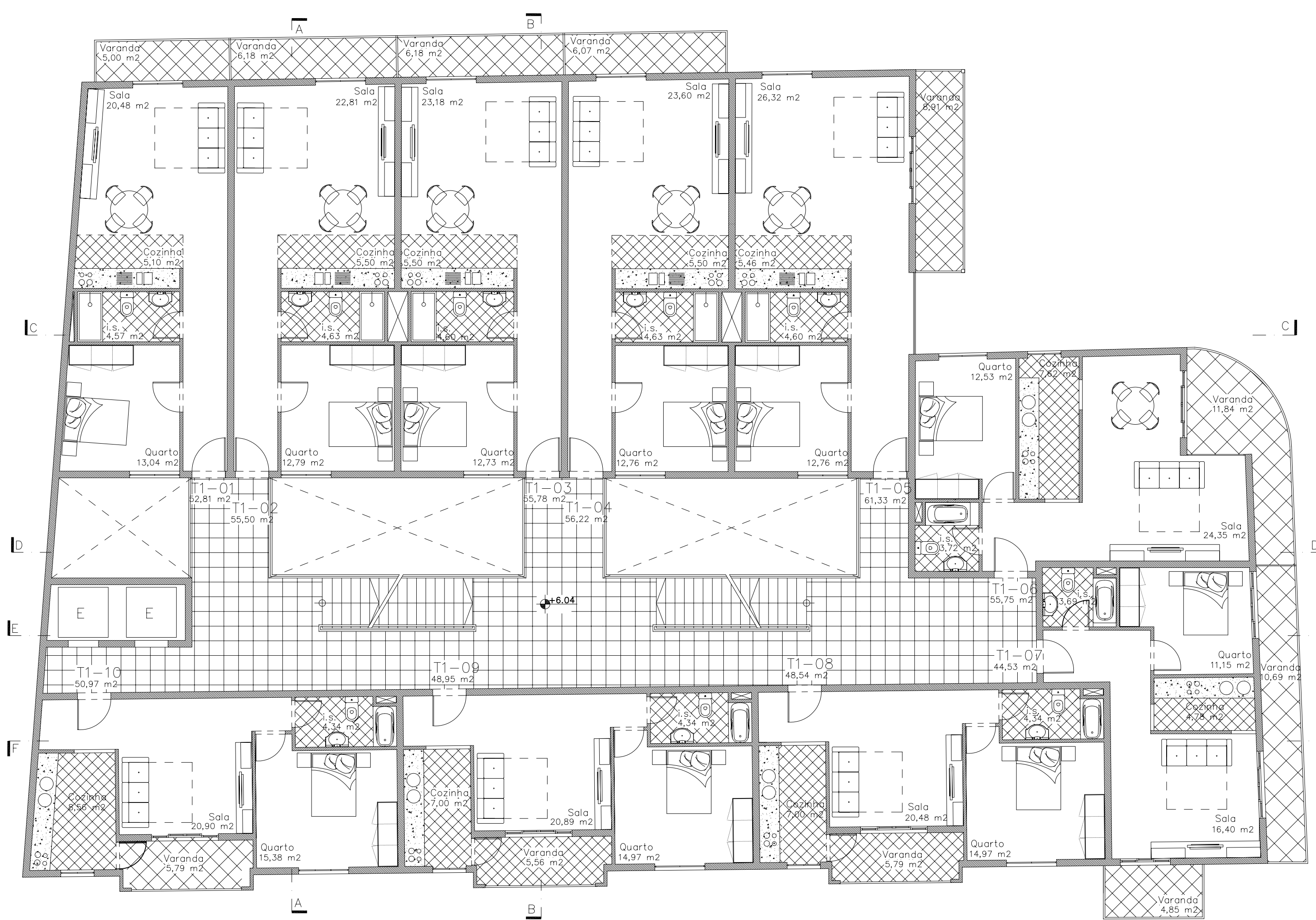
Planta Baixa do 1º Andar Esc. 1:100
